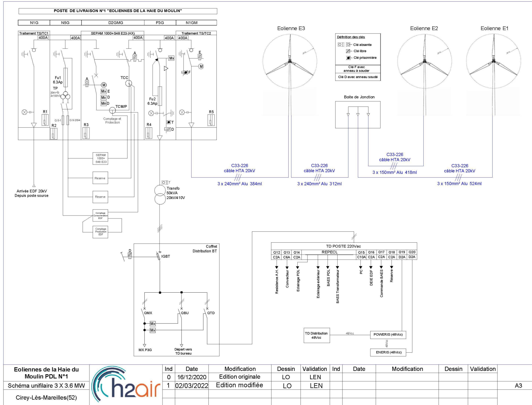
Figure 9 : Schéma unifilaire du PDL1 de la Haie du Moulin
