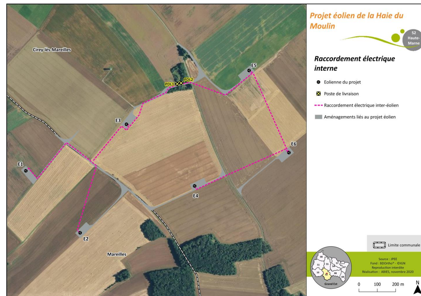
Carte 15 : Plan du raccordement inter-éolien et des postes de livraison
