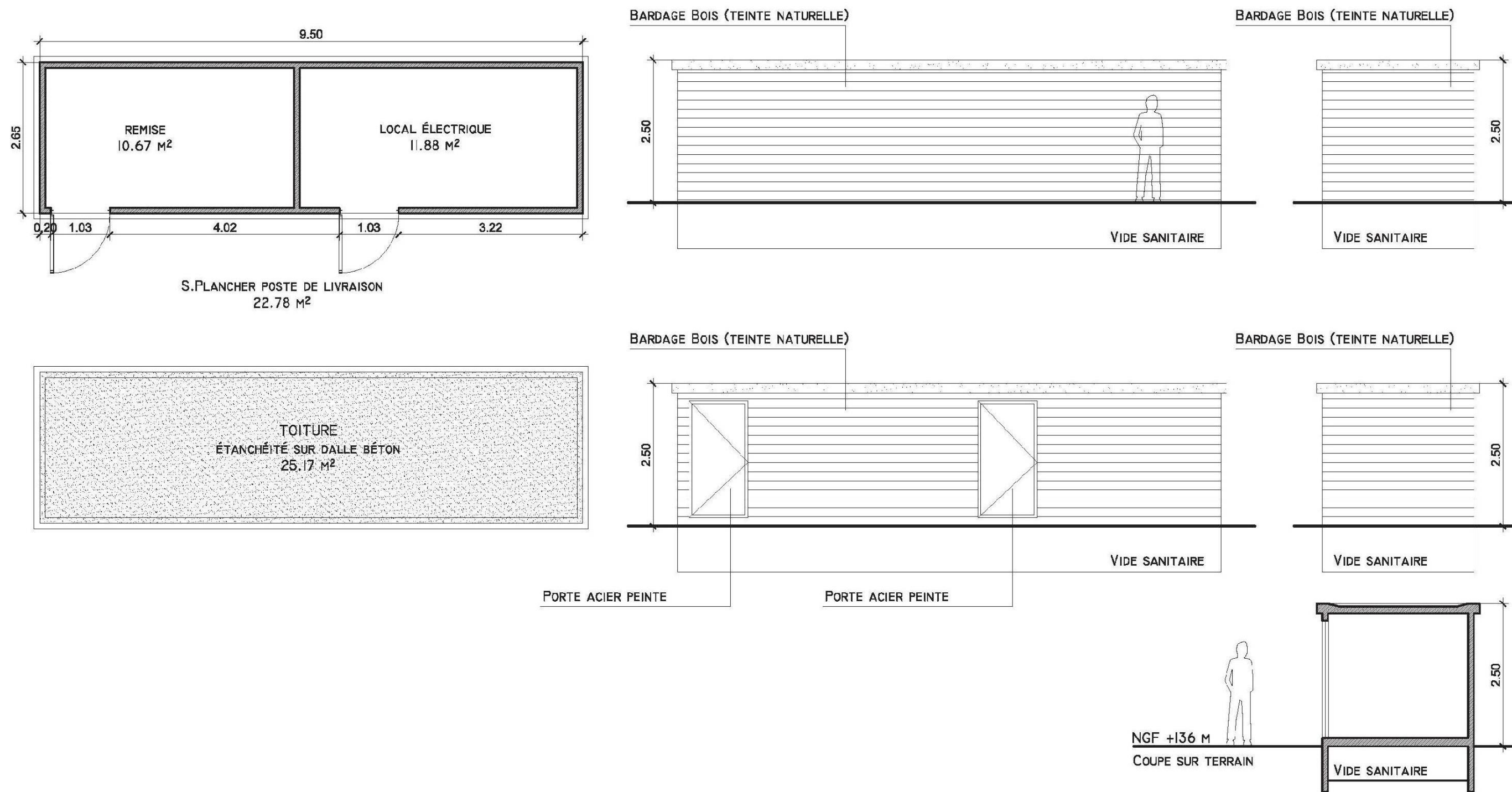
Figure 8 : Plan de masse des postes de livraison
