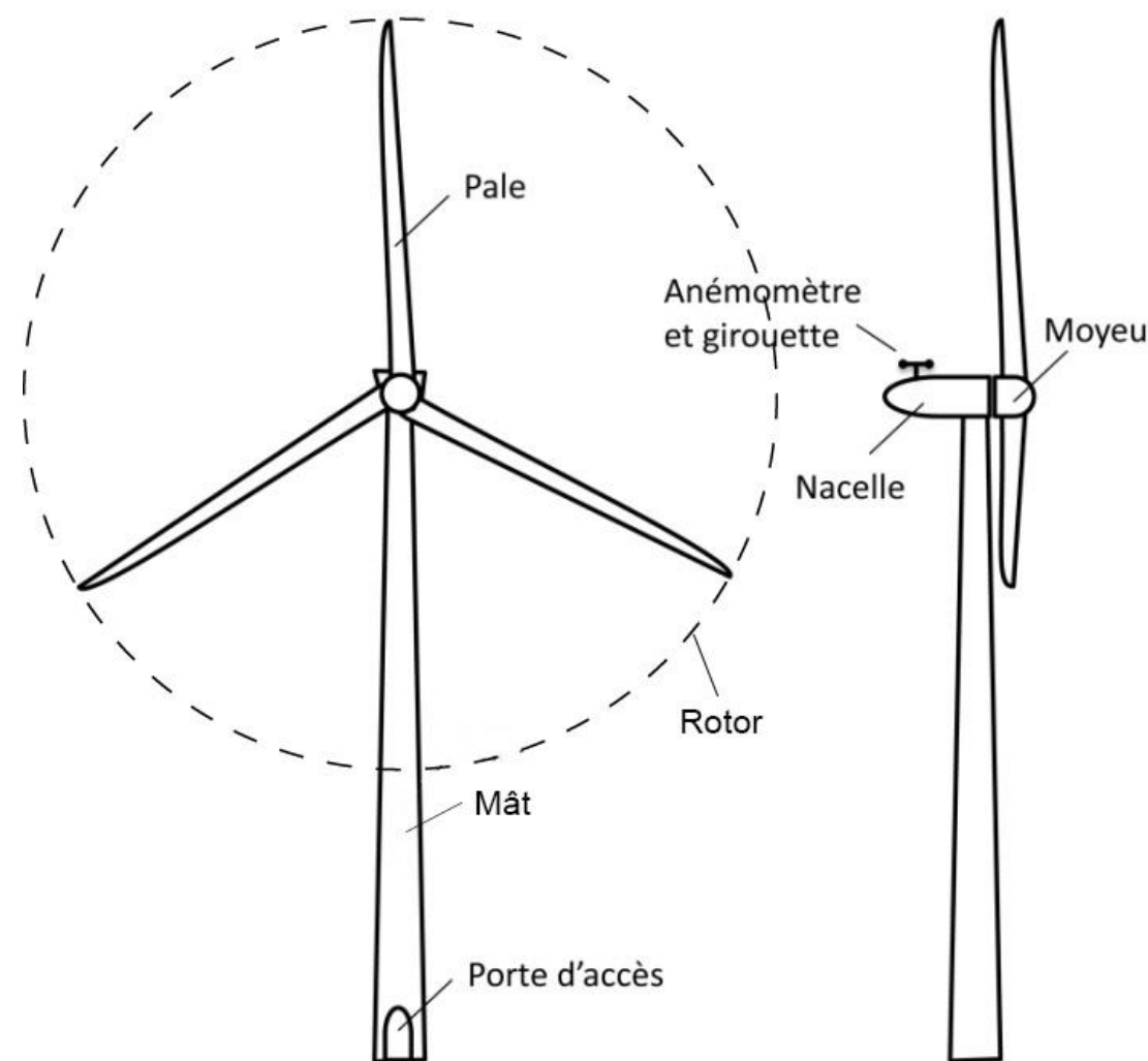
Figure 2 : Schéma simplifié d'un aérogénérateur
