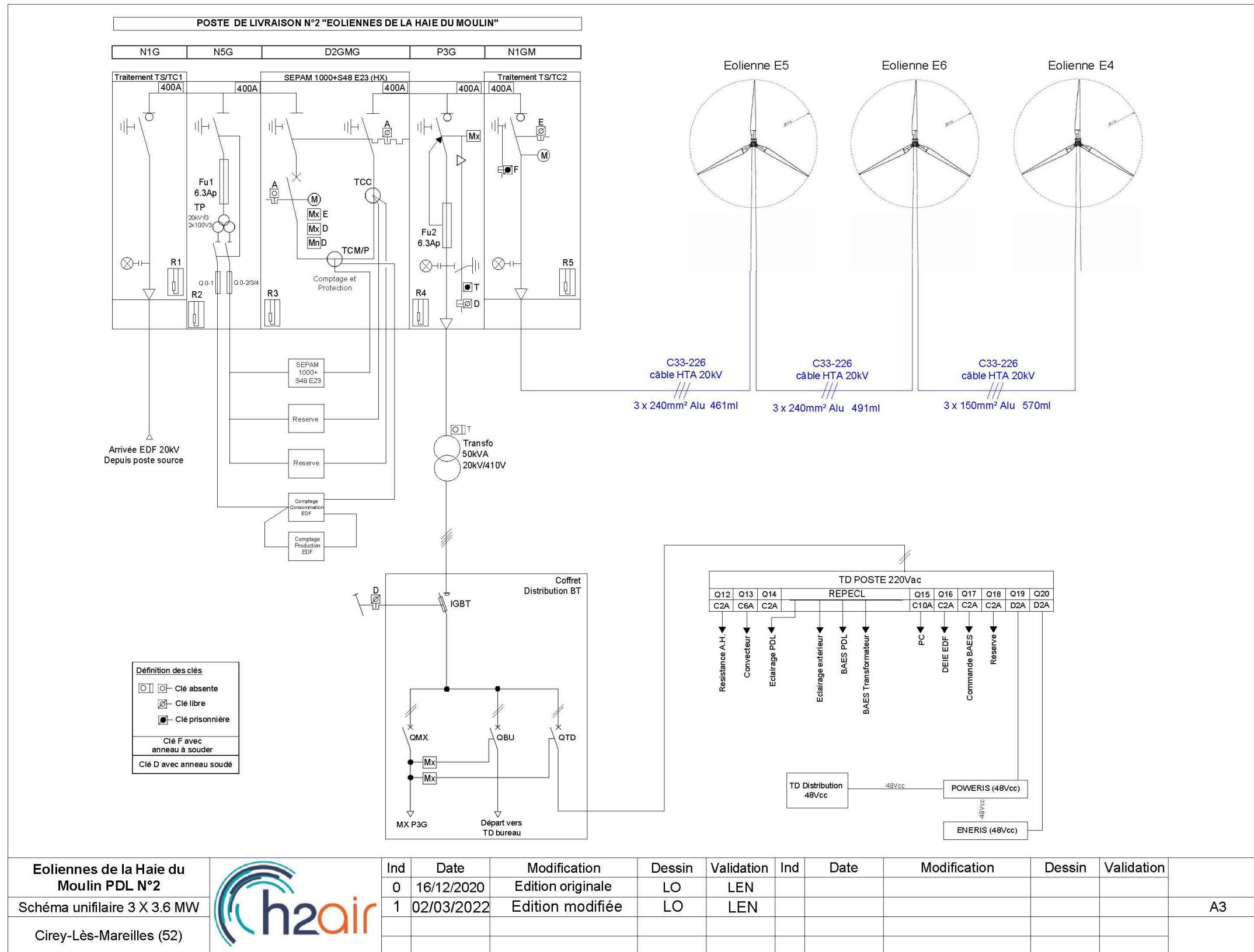
Figure 10 : Schéma unifilaire de la PDL2 de la Haie du Moulin
